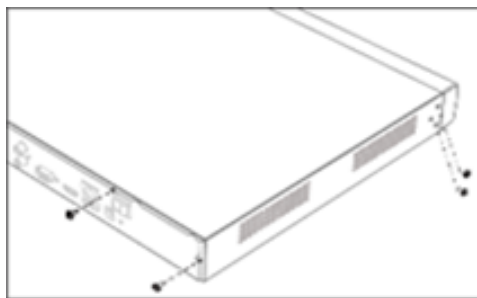
Abbildung 2-1 Abdeckung entfernen
