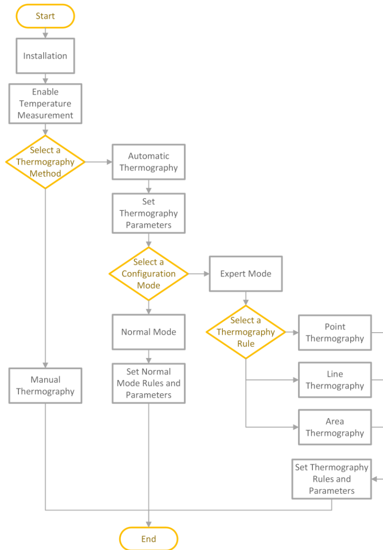
Abbildung 7-1 Flussdiagramm zur Konfiguration der Thermografie
