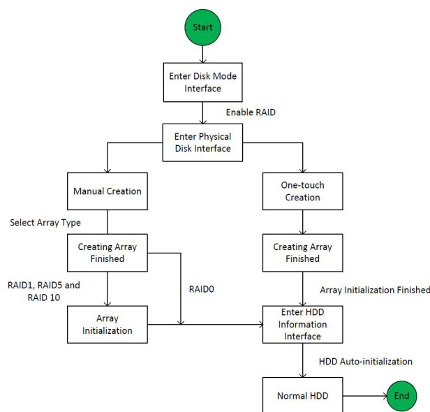
RAID-Prozessfluss
