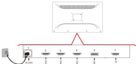
Abbildung 1-2 Anschlussleiste
