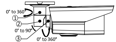
Abbildung 2-4 3-Achsenausrichtung
