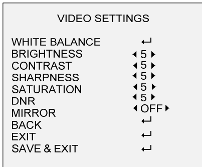
Abbildung 3-5 Bildeinstellungen
