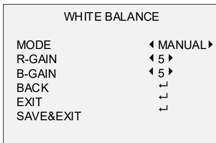
Abbildung 3-6 manueller Weißabgleich
