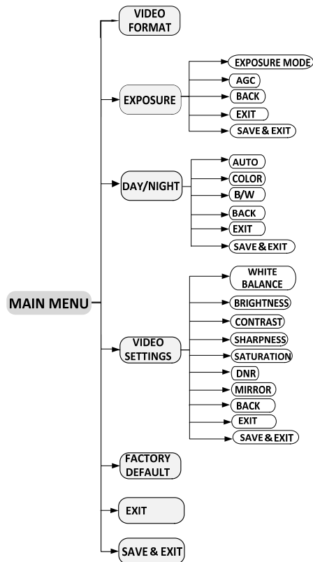
Abbildung 3-2 Hauptmenü
