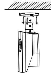
Abbildung 2-3 Kamera befestigen
