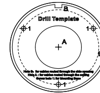
Abbildung 2-1 Bohrschablone
