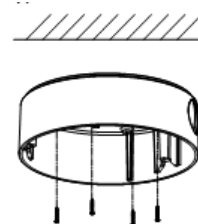
Abbildung 2-2 Montagesockel an der Wand/Decke befestigen
