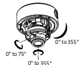
Abbildung 2-4 3-Achsenausrichtung
