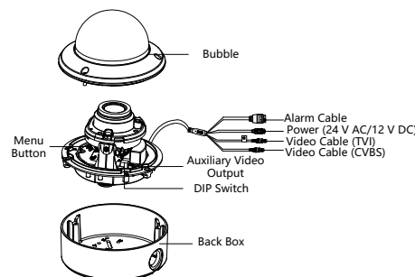
Abbildung 1-1 Kamerakomponenten
