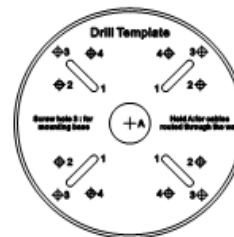
Abbildung 2-1 Bohrschablone
