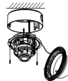
Abbildung 2-3 Kamera an Decke befestigen
