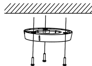
Abbildung 2-2 Montagesockel an der Wand/Decke befestigen
