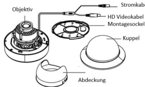
Abbildung 1-1 Kamerakomponenten
