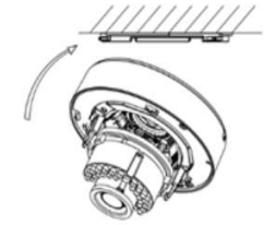
Abbildung 2-3 Kamera an Montagesockel befestigen
