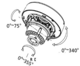
Abbildung 2-4 3-Achsenausrichtung
