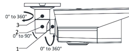
Abbildung 2-3 3-Achsenausrichtung
