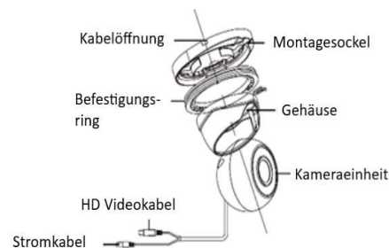
Abbildung 1-1 Kamerakomponenten
