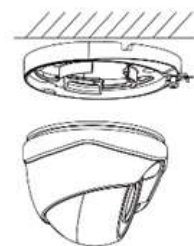
Abbildung 2-3 Kamera befestigen
