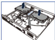
Abbildung 2-3 Festplatte festschrauben
