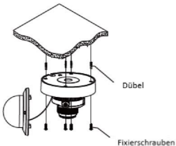
Abbildung 2-2 Kamera an Wand/Decke befestigen
