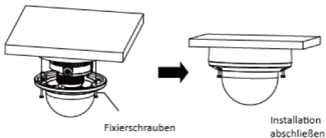
Abbildung 2-3 Kamera an Wand/Decke befestigen
