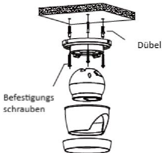
Abbildung 2-3 Kamera an Wand/Decke befestigen
