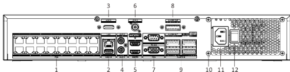
Abbildung 1-1 Anschlüsse auf der Rückseite
