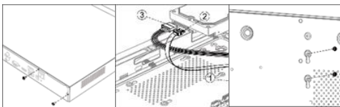
Abbildung 2-1 Abdeckung entfernen
