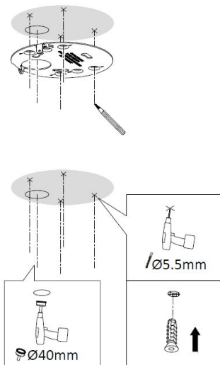
Abbildung 2-2 Installationsplatte
