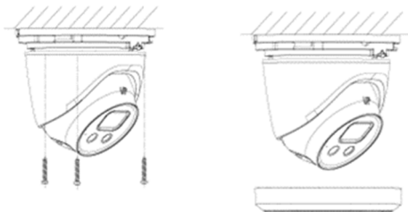
Abbildung 2-4 Kamera anbringen
