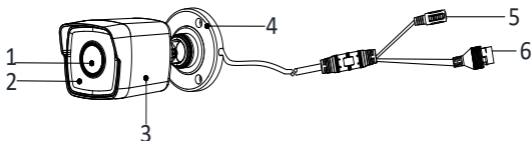
Abbildung 1-1 Kamera Überblick
