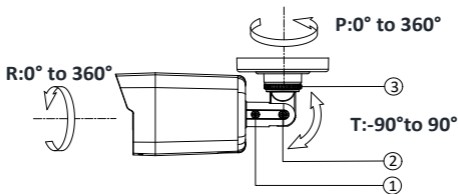
Abbildung 2-3 3-Achsen Einstellung
