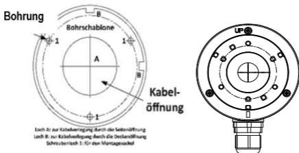
Abbildung 2-4 Bohrschablone
