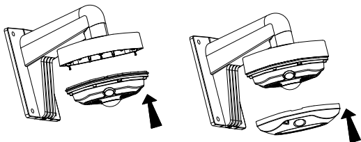
Abbildung 2-9 Installation der Kamera und der Abdeckung
