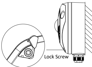
Abbildung 2-7 Abdeckung befestigen
