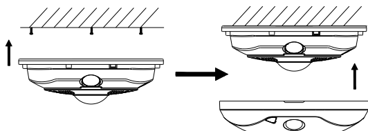
Abbildung 2-3 Wiederanbringen der Abdeckung
