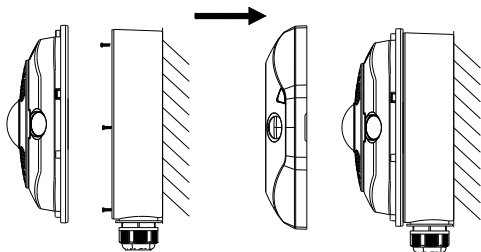
Abbildung 2-6 Anbringen der Kamera
