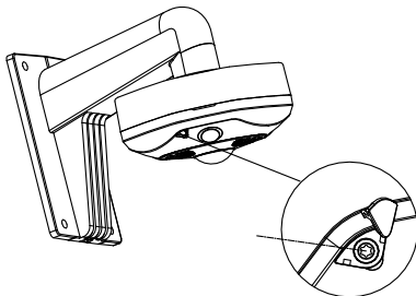
Abbildung 2-10 Abdeckung befestigen
