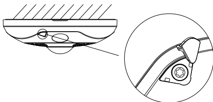
Abbildung 2-4 Kameraabdeckung befestigen
