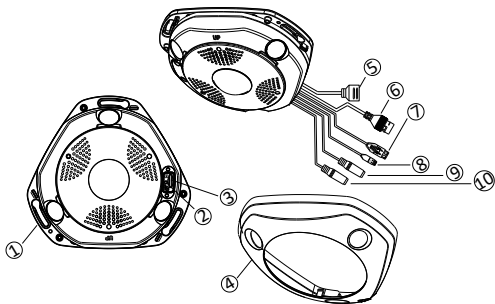
Abbildung 1-2 Öffnen des Gehäuses
