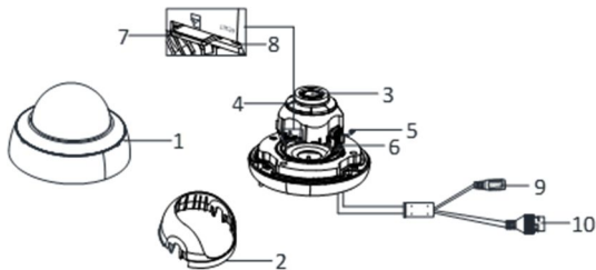
Abbildung 1-1 Kamera Übersicht
