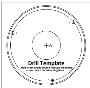
Abbildung 2-3 Bohrschablone
