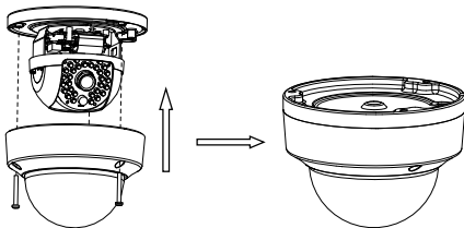
Abbildung 2-9 Kuppel wieder befestigen
