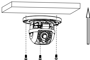
Abbildung 2-5 Befestigung des Montagesockels
