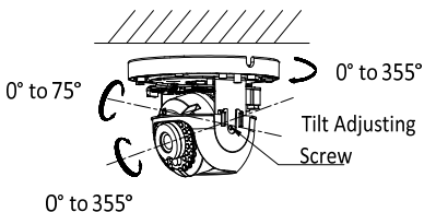
Abbildung 2-7 Kamera 3-Achsen-Einstellung
