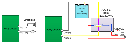
Abbildung 1-3 Alarmausgang
