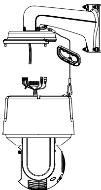
Abbildung 2.5 Sicherungsseil anbringen
