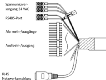
Abbildung 1-2 Kabelübersicht
