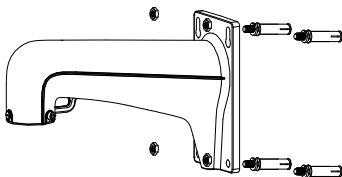
Abbildung 2-3 Wandhalterung
