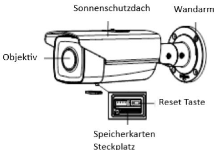
Abbildung 1-1 Überblick über die Kamera
