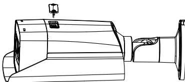
Abbildung 2-1 Abnehmen der Abdeckung des Speicherkartensteckplatzes
