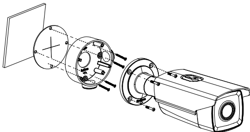
Abbildung 2-5 Anbringen des Adapters
