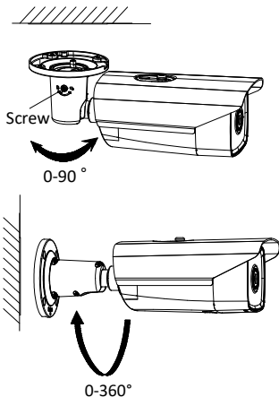
Abbildung 2-6 Anpassen des Blickwinkels
