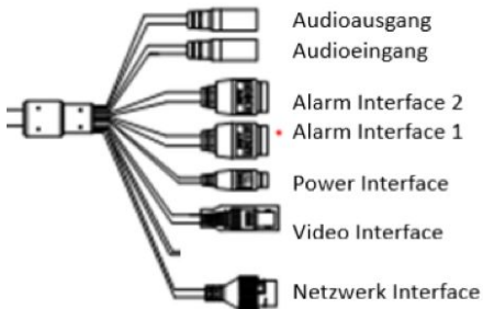
Abbildung 1-2 Überblick über den Kabelbaum
