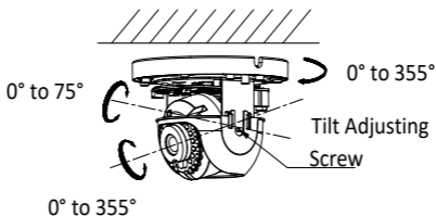
Abbildung 2-7 Kamera 3-Achsen-Einstellung
