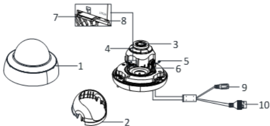
Abbildung 1-1 Kamera Übersicht
