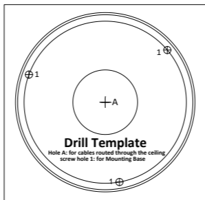
Abbildung 2-3 Bohrschablone
