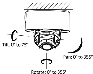
Abbildung 2-7 3-Achsen-Einstellung
