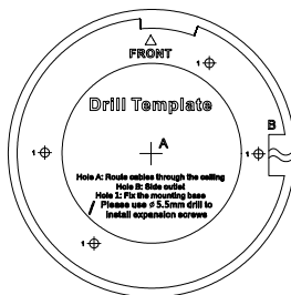
Abbildung 2-3 Bohrschablone
