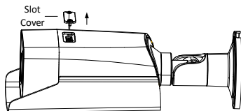
Abbildung 2-1 Speicherkartensteckplatz freilegen
