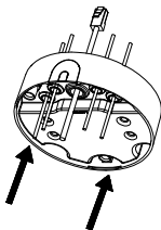
Abbildung 2-8 Führen des Kabels durch die Anschlussdose
