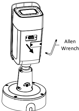
Abbildung 2-1 Abnehmen der Abdeckung des Speicherkartensteckplatzes
