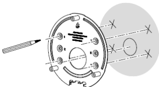
Abbildung 2-4 Bohren Sie Löcher in die Wand / Decke
