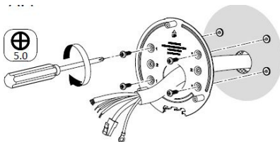
Abbildung 2-5 Anbringen des Adapters
