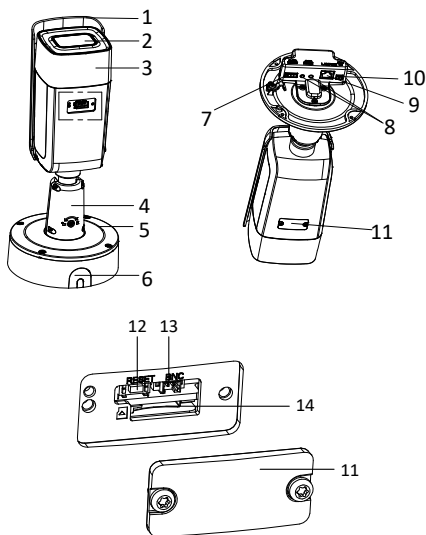
Abbildung 1-1 Überblick über die Kamera
