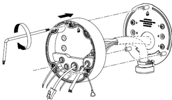
Abbildung 2-9 Befestigen der Anschlussdose
