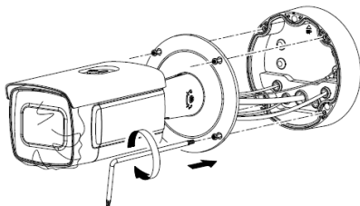
Abbildung 2-11 Befestigen der Kamera
