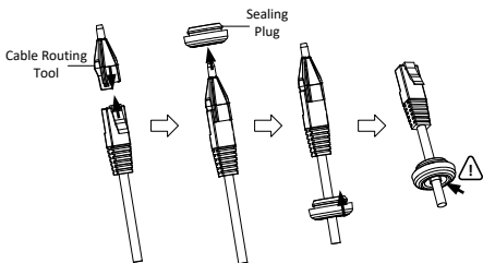
Abbildung 2-7 Führen des RJ45-Netzkabels durch den Verschlussstopfen
