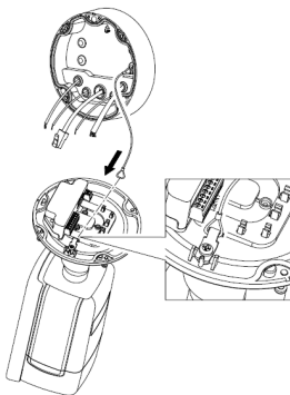
Abbildung 2-10 Anhängen der Kamera an die Anschlussdose
