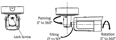
Abbildung 2-12 Anpassen des Blickwinkels
