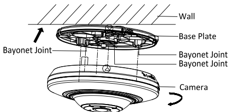
Abbildung 2-4 Kamera anbringen
