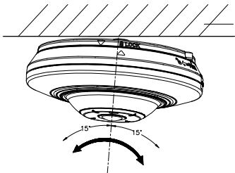
Abbildung 2-6 Blickwinkel anpassen
