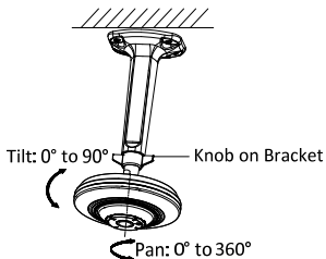
Abbildung 2-19 Blickwinkel anpassen
