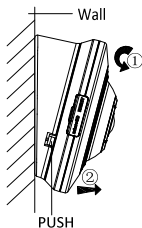
Abbildung 2-11 Kamera abnehmen
