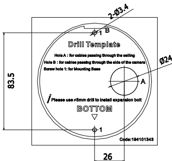
Abbildung 2-7 Bohrschablone
