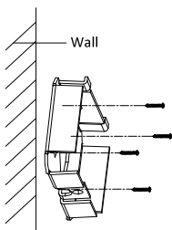
Abbildung 2-15 Montagesockel befestigen
