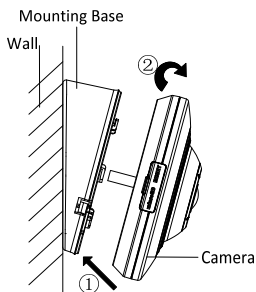
Abbildung 2-9 Kamera befestigen
