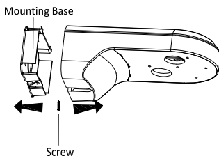
Abbildung 2-12 Halterung demontieren
