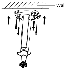
Abbildung 2-17 Halterung befestigen
