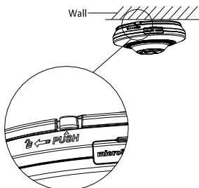
Abbildung 2-5 Kamera abnehmen
