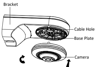
Abbildung 2-14 Kamera befestigen
