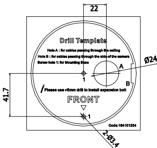
Abbildung 2-2 Bohrschablone
