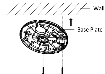
Abbildung 2-3 Montageplatte befestigen
