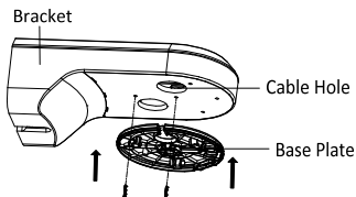
Abbildung 2-13 Montageplatte befestigen
