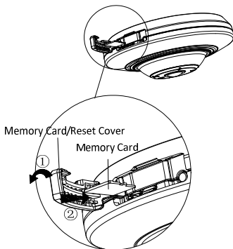
Abbildung 2-1 Speicherkarte einlegen
