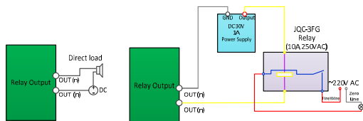
Abbildung 1-3 Alarmausgang
