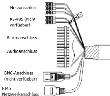
Abbildung 1-2 Kabelübersicht
