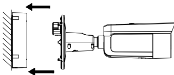
Abbildung 2-10 Befestigen der Kamera
