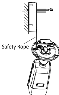
Abbildung 2-9 Anhaken der Kamera an die Anschlussdose
