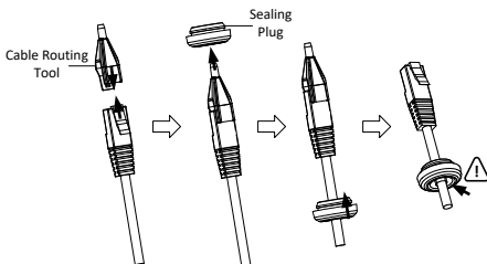
Abbildung 2-7 Führen des RJ45-Netzwerkkabels durch den Verschlussstopfen
