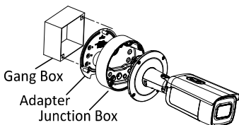
Abbildung 2-13 Montage mit einer Unterputzdose
