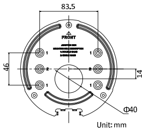
Abbildung 2-4 Bohren Sie Löcher in die Wand / Decke
