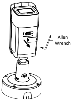
Abbildung 2-1 Abnehmen der Abdeckung des Speicherkartensteckplatzes
