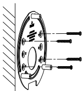
Abbildung 2-5 Anbringen des Adapters
