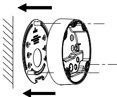
Abbildung 2-9 Befestigen der Anschlussdose
