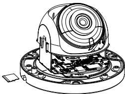
Abbildung 2-2 Speicherkarte einsetzen
