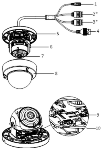
Abbildung 1-1 Kameraübersicht
