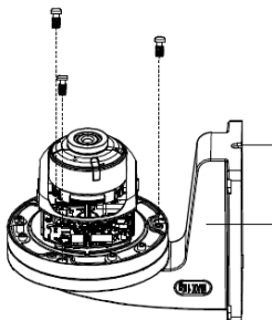
Abbildung 2-9 Kamera an Wandhalterung befestigen
