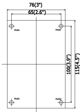
Abbildung 2-8 Bohrungen markieren
