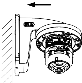
Abbildung 2-10 Wandhalterung anbringen
