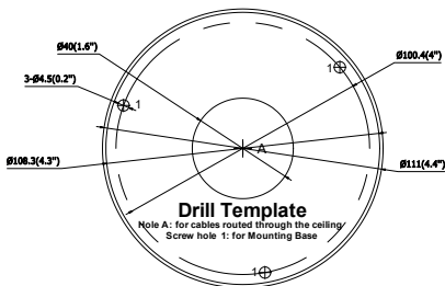
Abbildung 2-3 Bohrschablone
