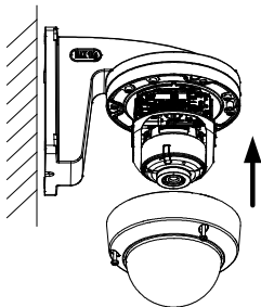
Abbildung 2-11 Kuppel aufsetzen
