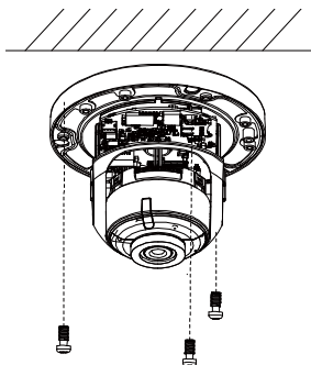
Abbildung 2-5 Kamerasockel besfestigen
