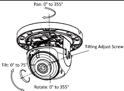
Abbildung 2-6 Blickwinkel einstellen
