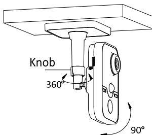
Abbildung 2-6 Kamerawinkel anpassen.
