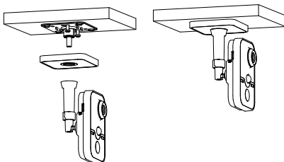
Abbildung 2-5 Kamera befestigen
