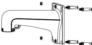
Abbildung 2-3 Wandhalterung
