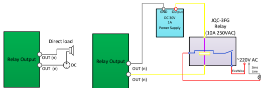
Abbildung 1-3 Alarmausgang
