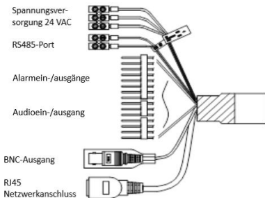
Abbildung 1-2 Kabelübersicht
