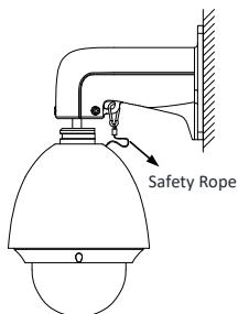
Abbildung 2-4 Sicherungsseil anbringen
