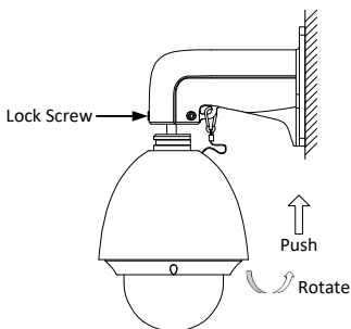
Abbildung 2-5 Kamera befestigen
