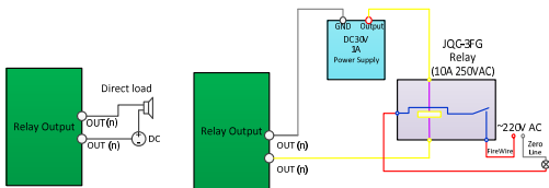
Abbildung 1-2 Alarmausgang
