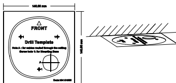
Abbildung 2-5 Befestigen der Bohrschablone
