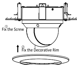
Abbildung 2-14 Abdeckring aufsetzen
