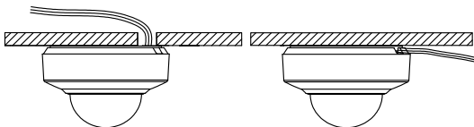
Abbildung 2-4 Kabelführung der Kamera
