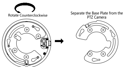
Abbildung 2-10 Kamera von Sockel lösen
