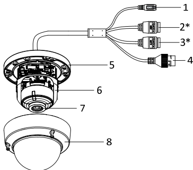
Abbildung 1-1 Schnittstellen und Kameraübersicht
