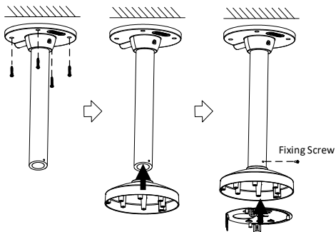
Abbildung 2-15 Abgehängene Halterung montieren
