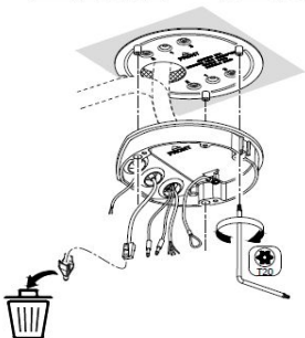
Abbildung 2-7 Kabel durch die Anschlussdose verlegen
