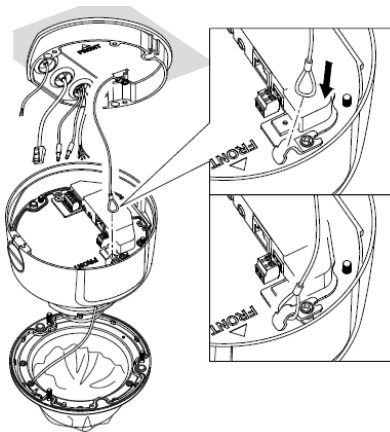
Abbildung 2-8 Anschlussdose montieren
