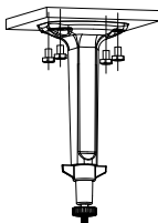
Abbildung 2-2 Halterung montieren
