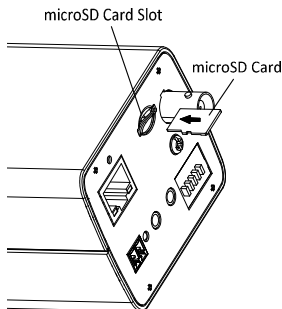
Abbildung 2-1 Speicherkarte einstecken
