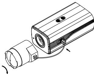
Abbildung 2-1 Objektiv anbringen
