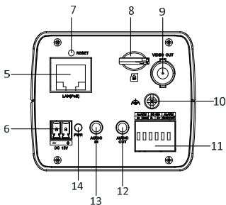
Abbildung 1-1 Kamera Übersicht
