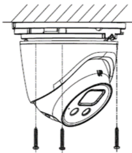
Abbildung 2.4 Kamerabasis befestigen
