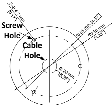
Abbildung 2.2 Bohrschablone
