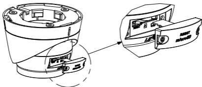
Abbildung 2.1 Abdeckung lösen
