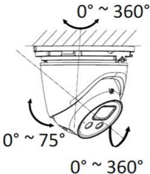
Abbildung 2.6 Betrachtungswinkel einstellen
