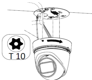
Abbildung 2.3 Kamera zerlegen
