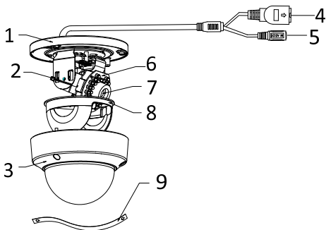
Abbildung 1-1 Kamera Übersicht
