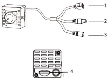
Abbildung 1-1 Kamera Überblick
