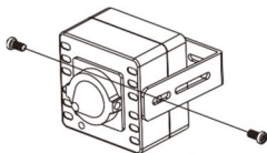
Abbildung 2-2 Kamera befestigen
